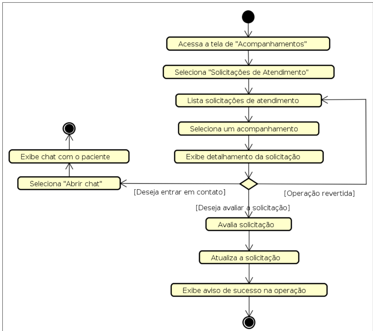
Figura 16 – Diagrama de atividade - Avaliar solicitação de acompanhamento
