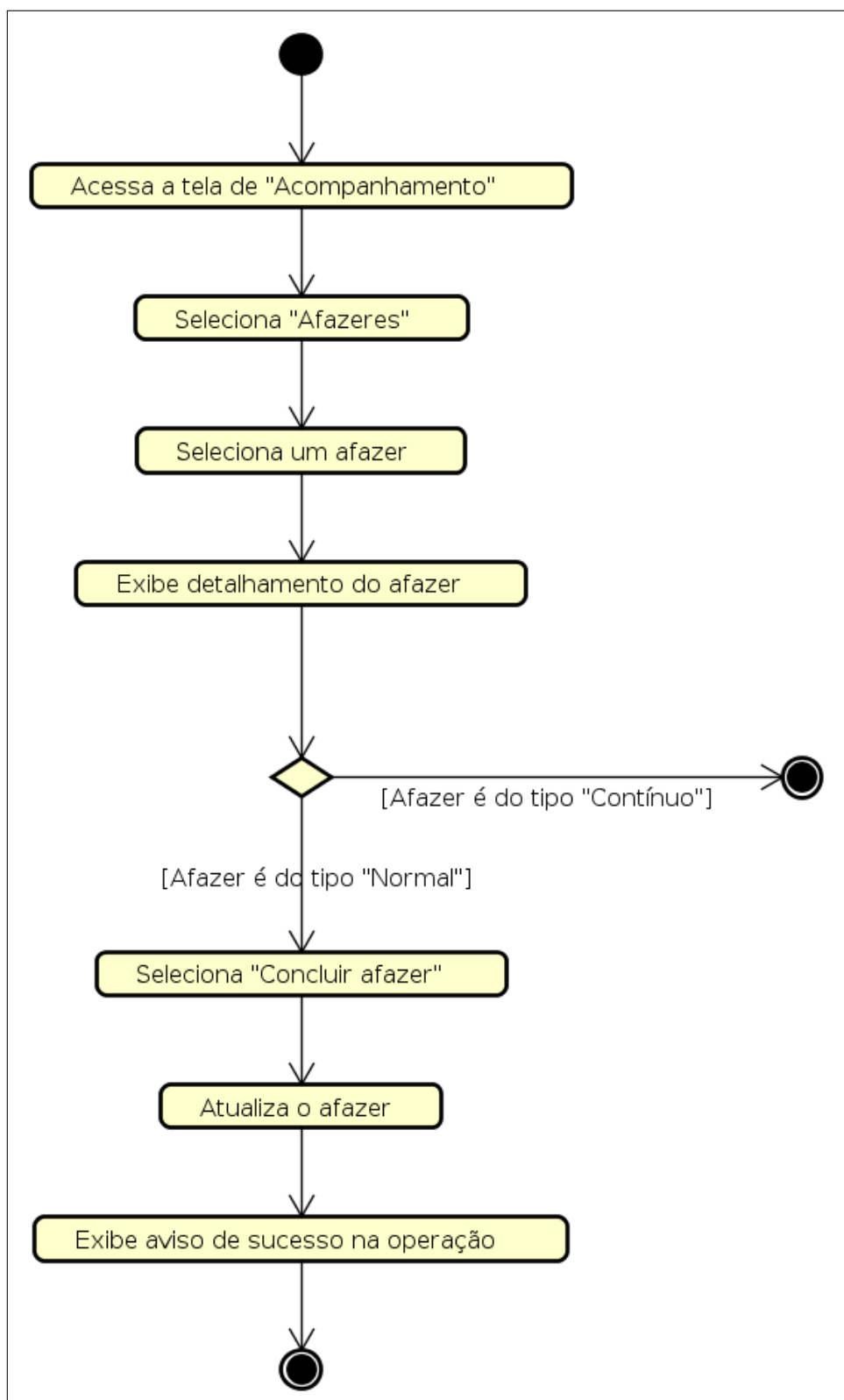
Figura 18 – Diagrama de atividade - Registrar afazer
