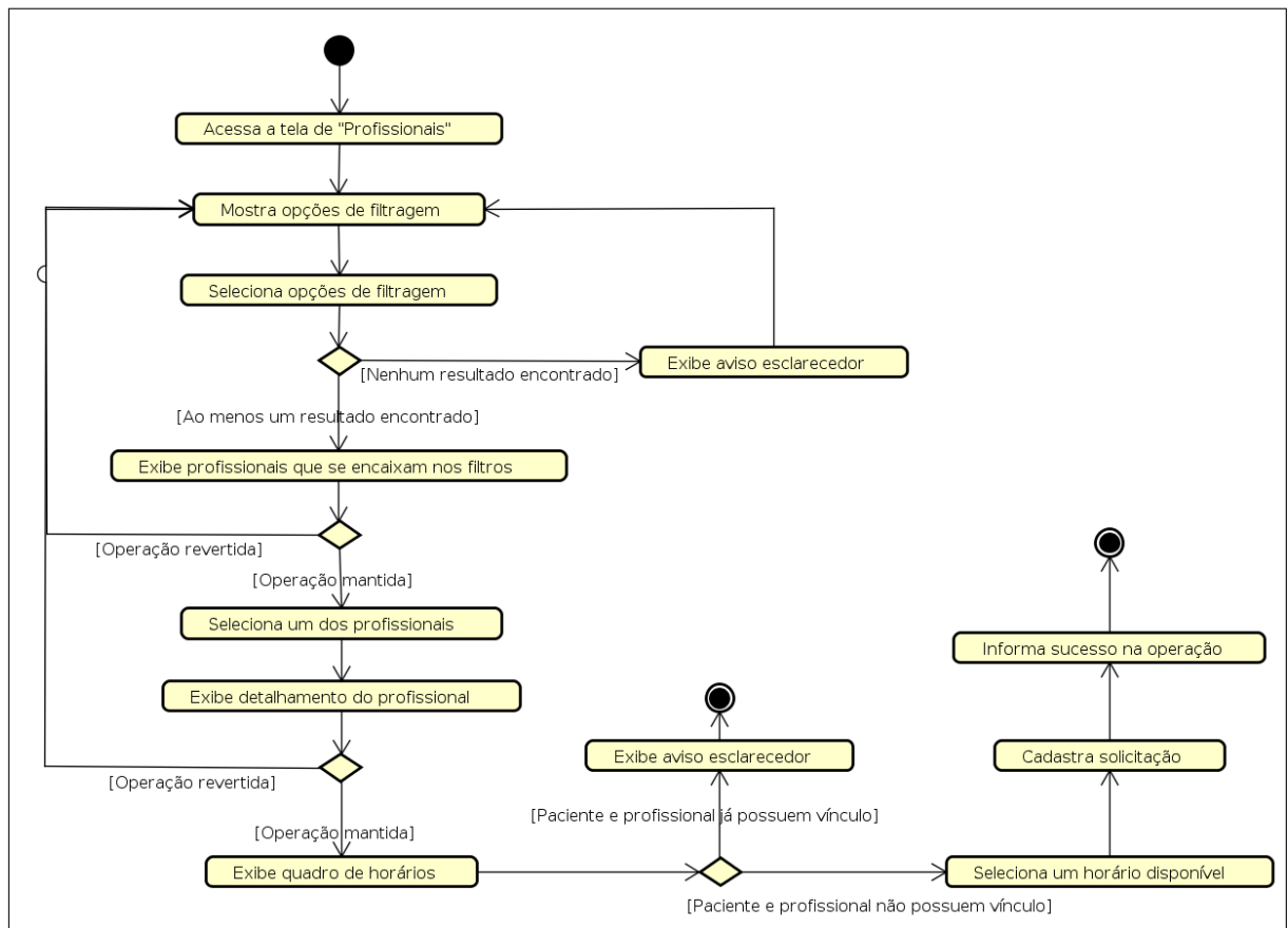
Figura 15 – Diagrama de atividade - Solicitação de acompanhamento
