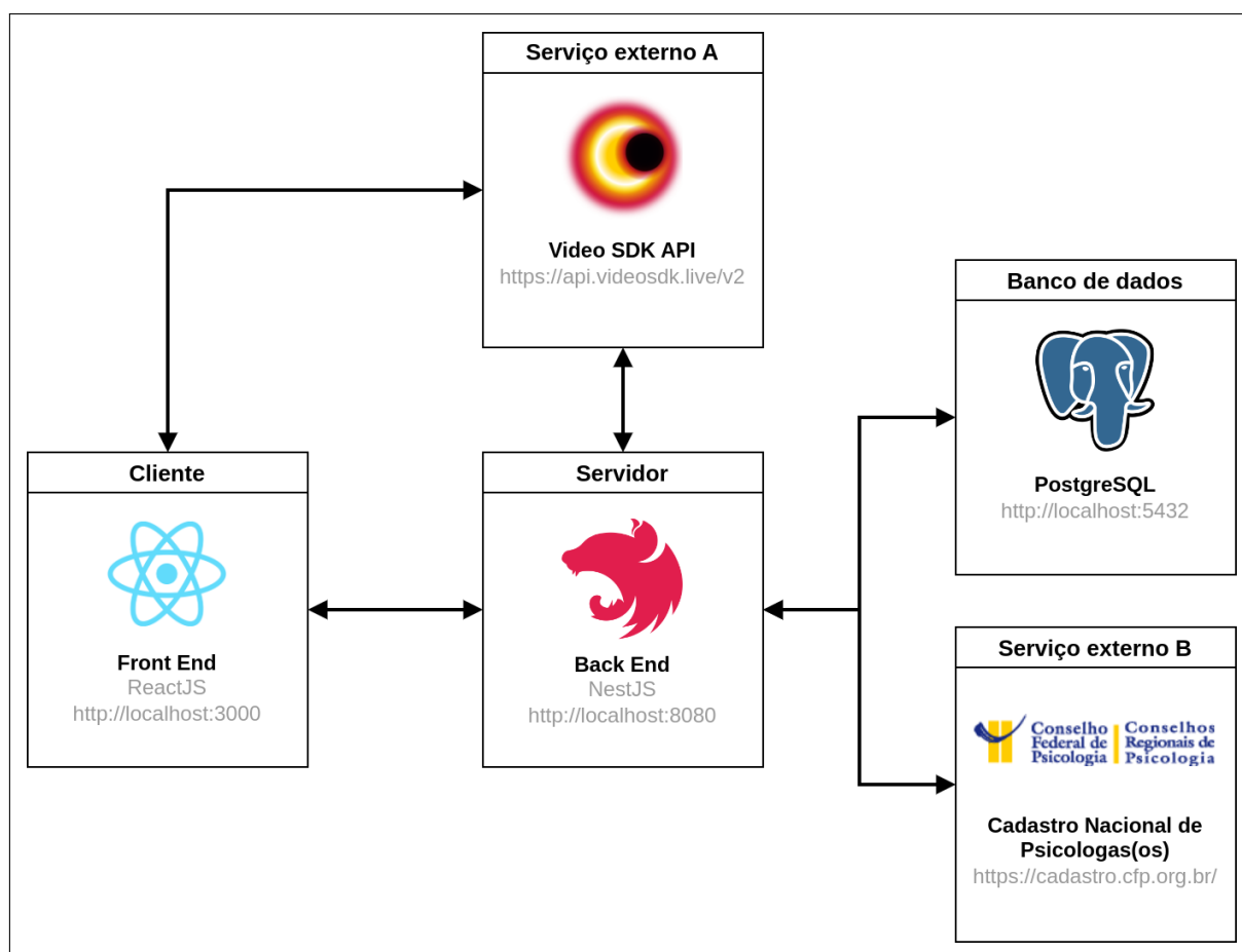
Figura 20 – Diagrama da arquitetura do sistema
