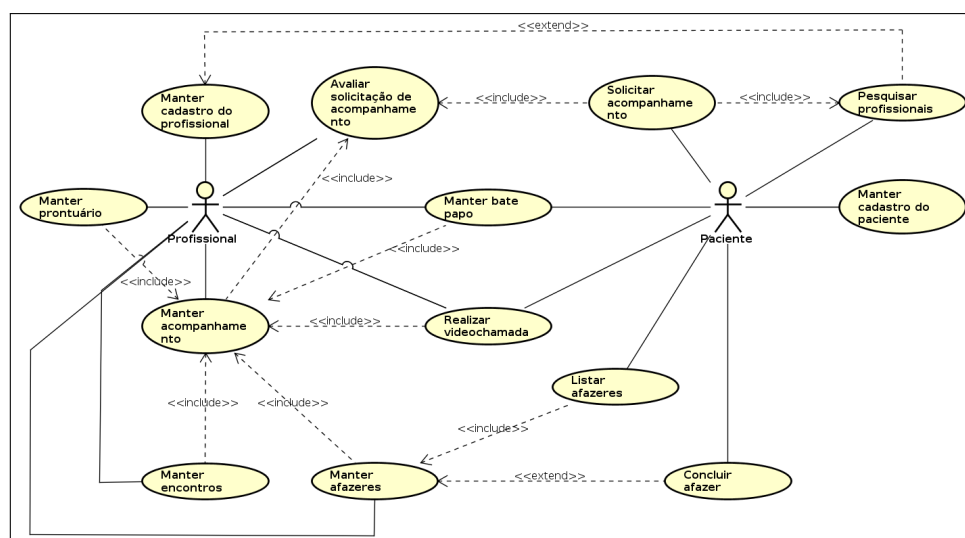
Figura 13 – Diagrama de caso de uso
