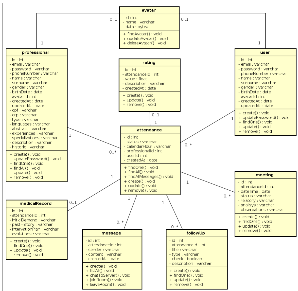
Figura 14 – Diagrama de classes
