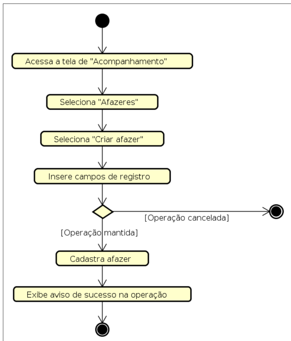
Figura 19 – Diagrama de atividade - Concluir afazer
