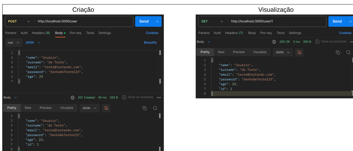
Figura 21 – Consumo da API de exemplo
