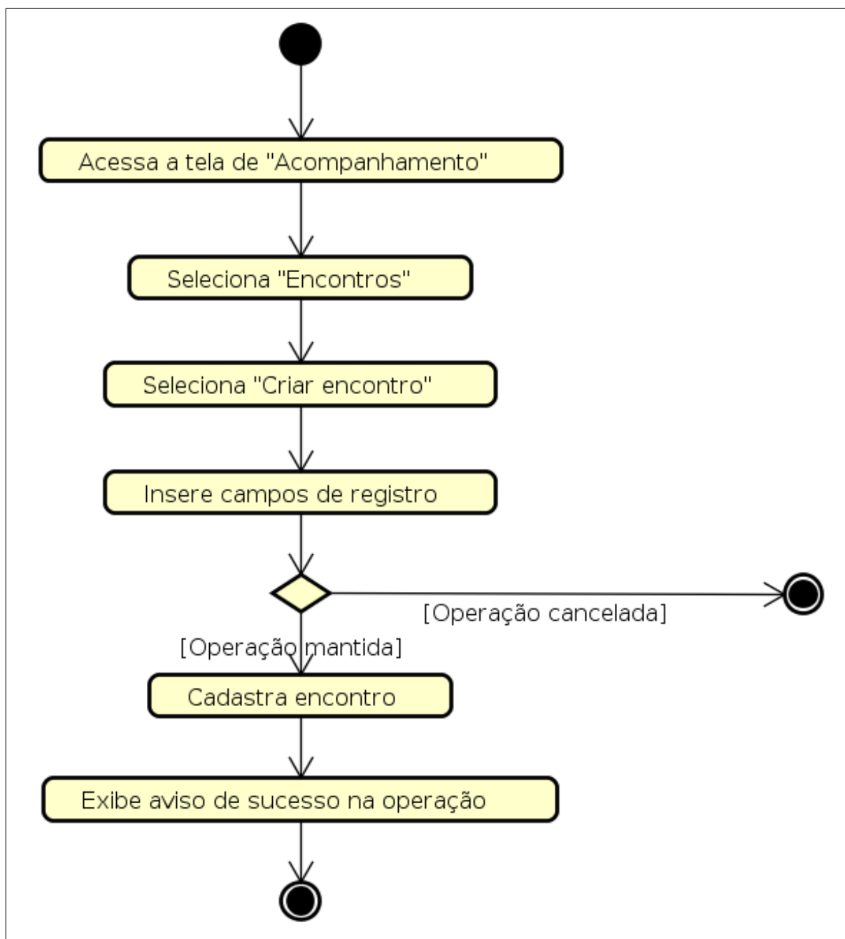
Figura 17 – Diagrama de atividade - Registrar encontro
