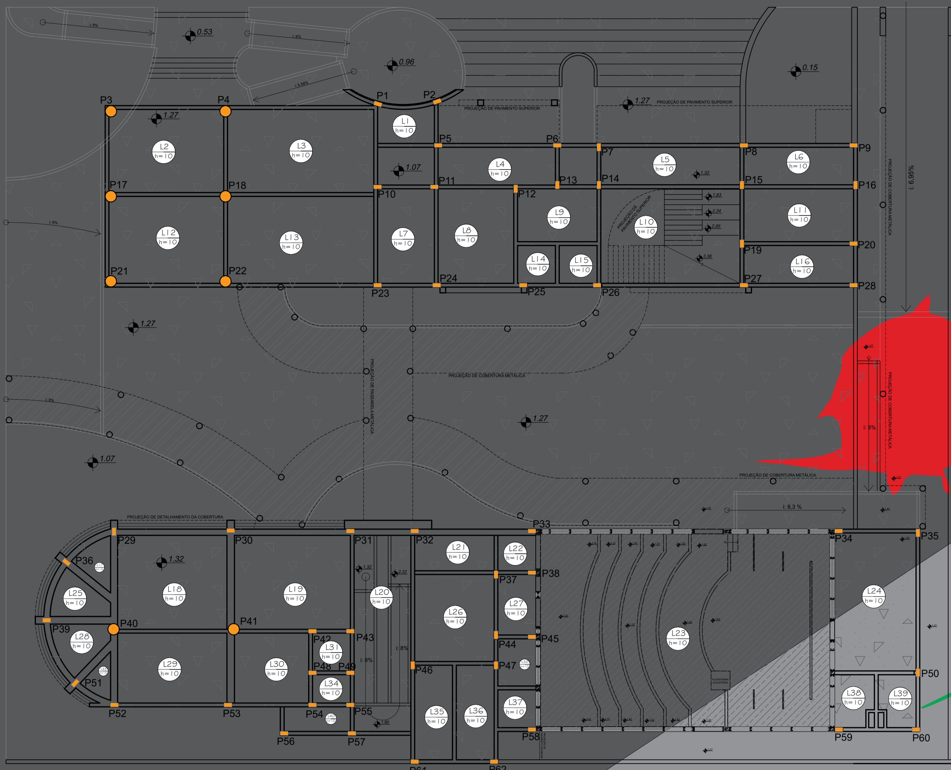
PLANTA ESTRUTURAL TÉRREO
