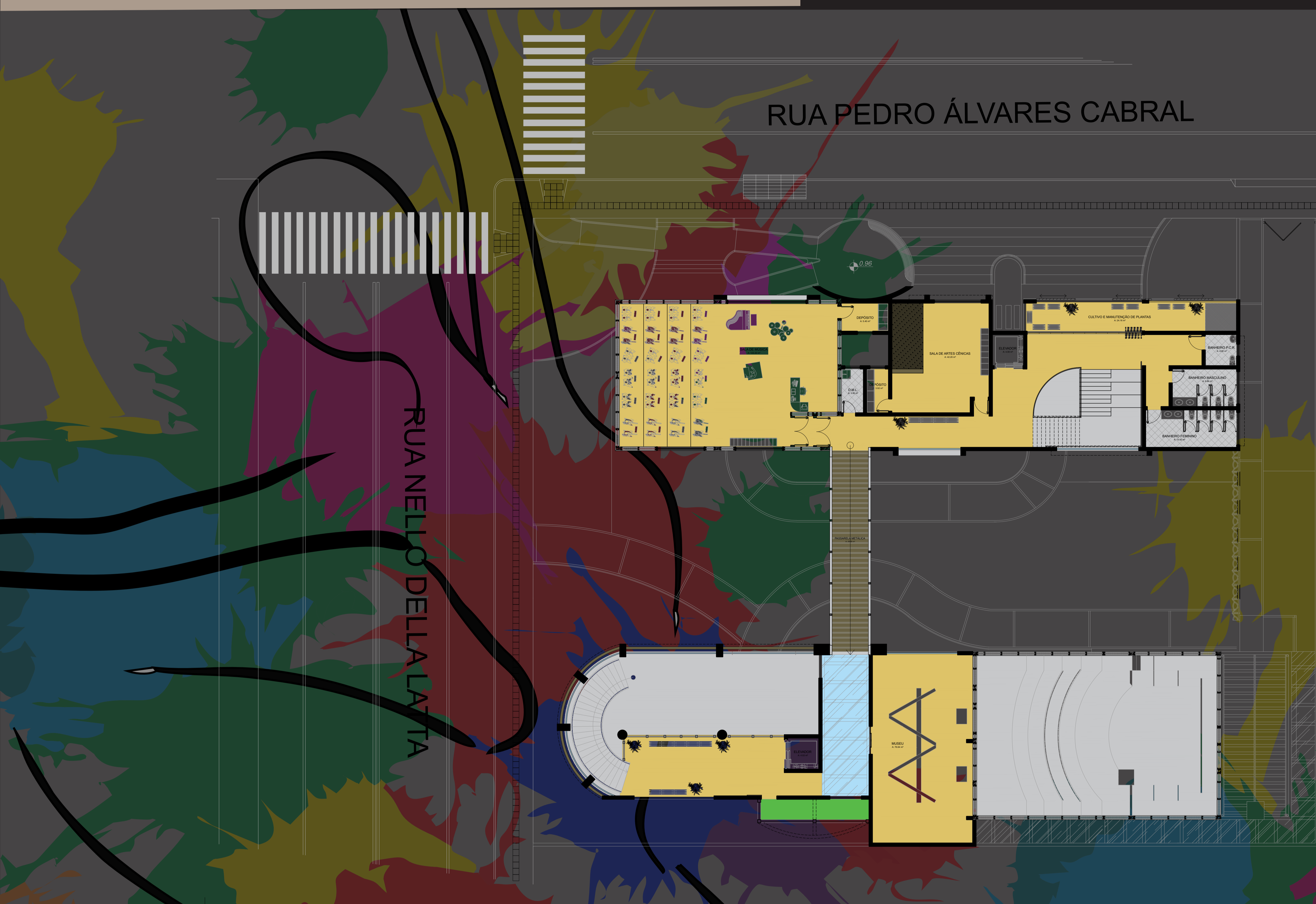
PLANTA HUMANIZADA 1º PAV. ESCALA 1:125
