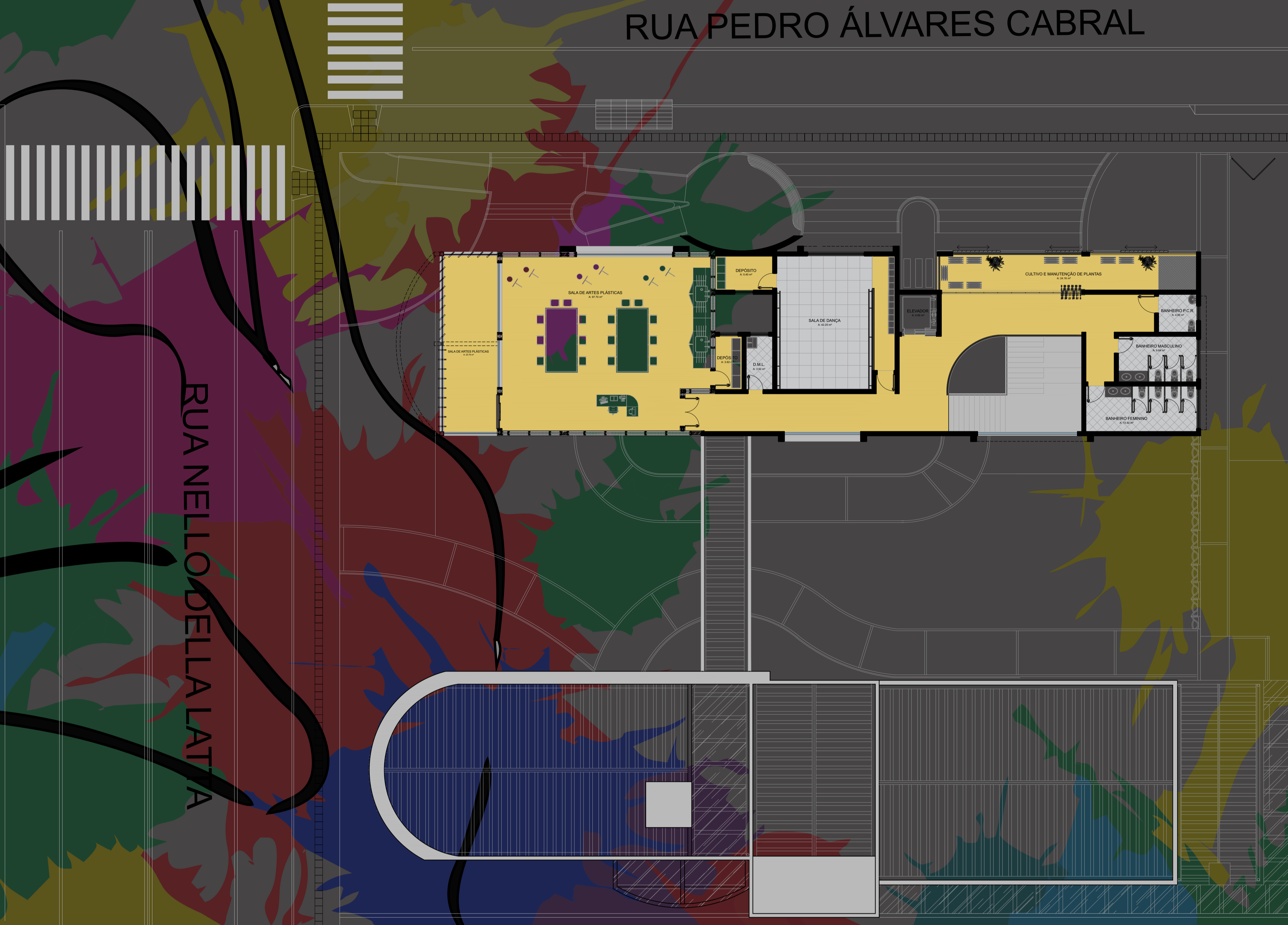
PLANTA HUMANIZADA 2º PAV. ESCALA 1:125
