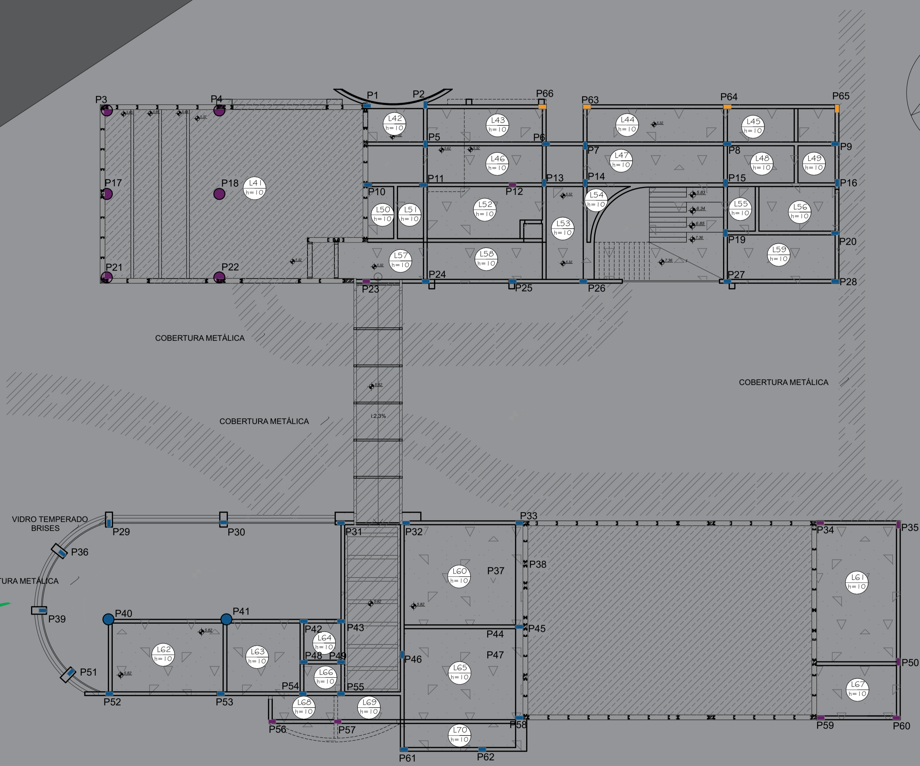
PLANTA ESTRUTURAL 1º PAV.
